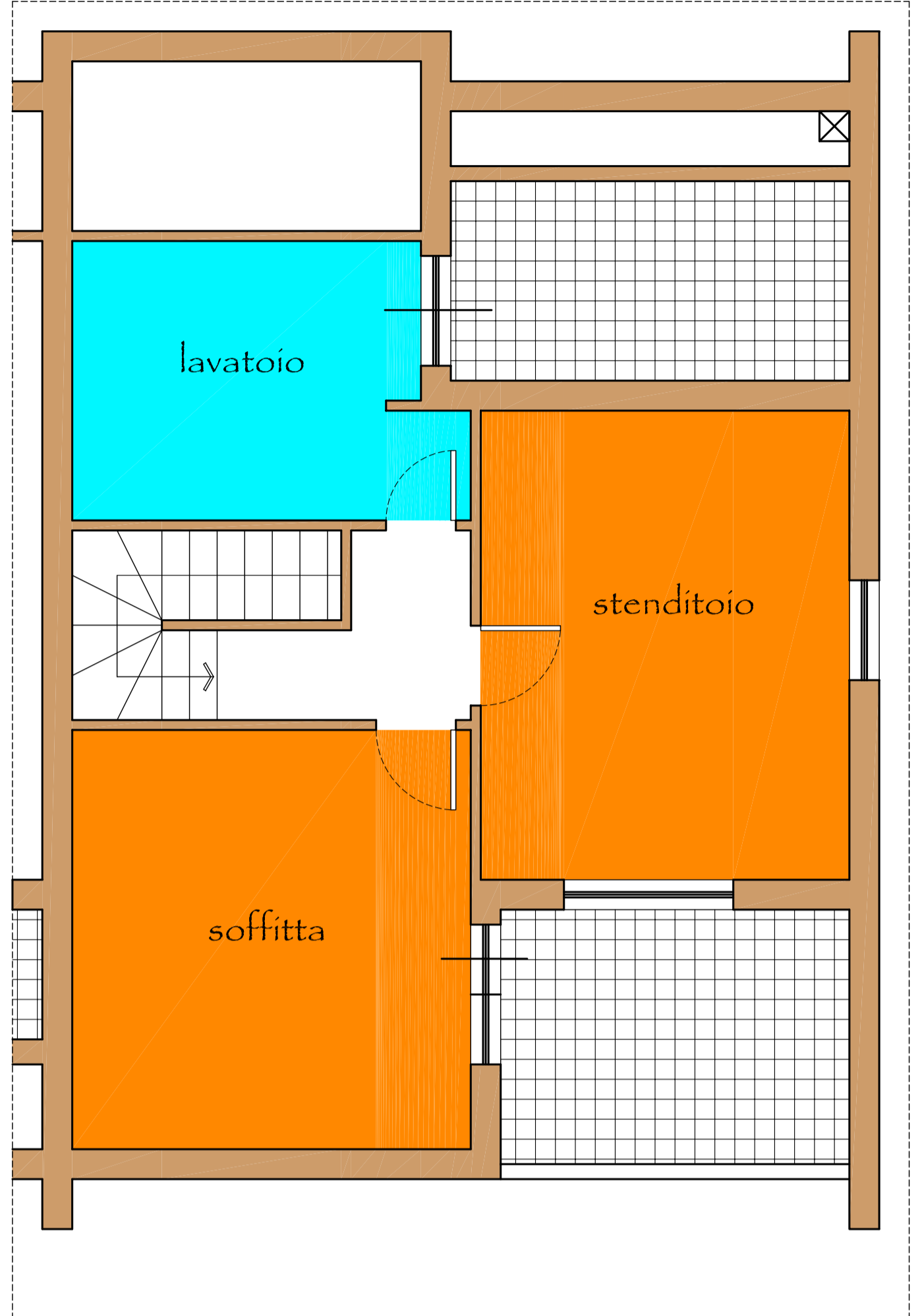
Piano sottotetto Superficie 63 mq.
