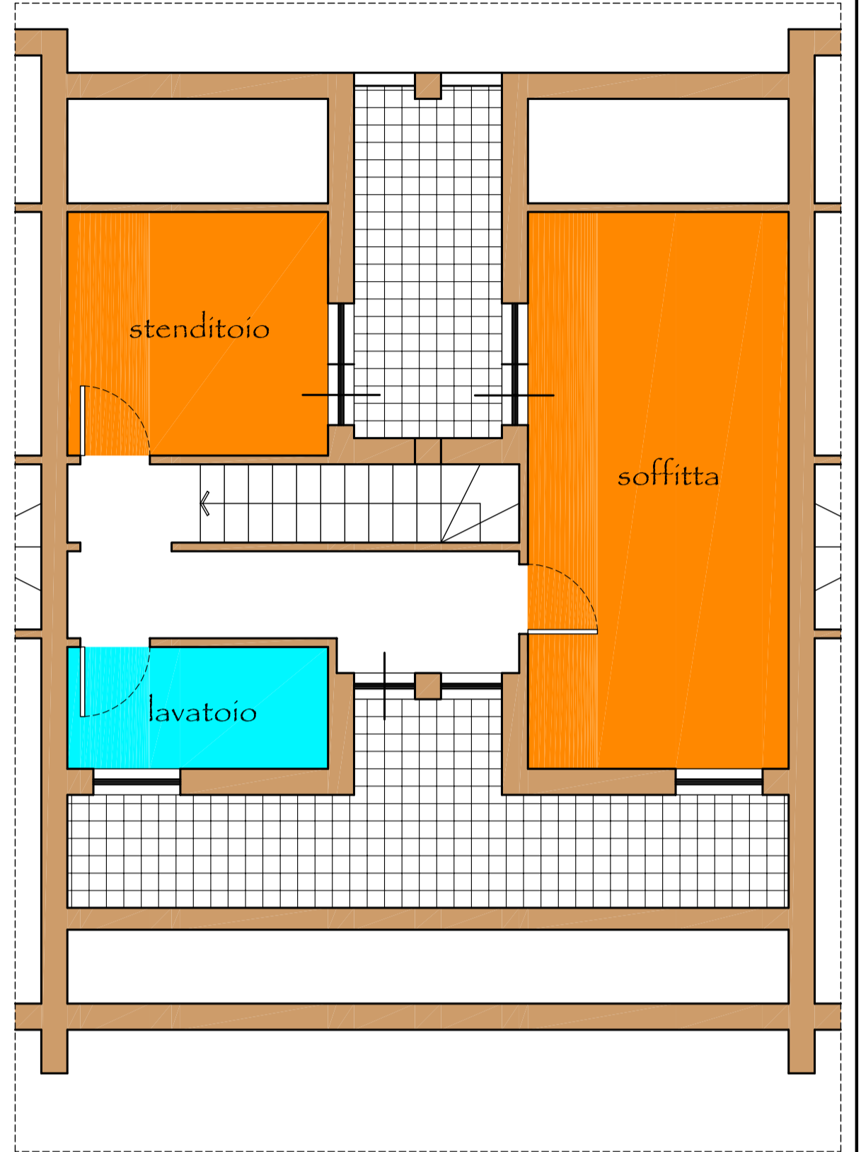
Piano sottotetto Superficie 54 mq.
